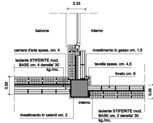
PARTICOLARE B
