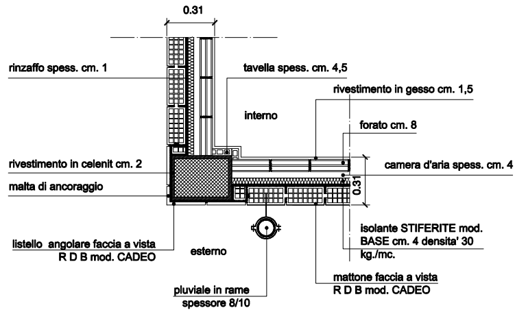
PARTICOLARE A
