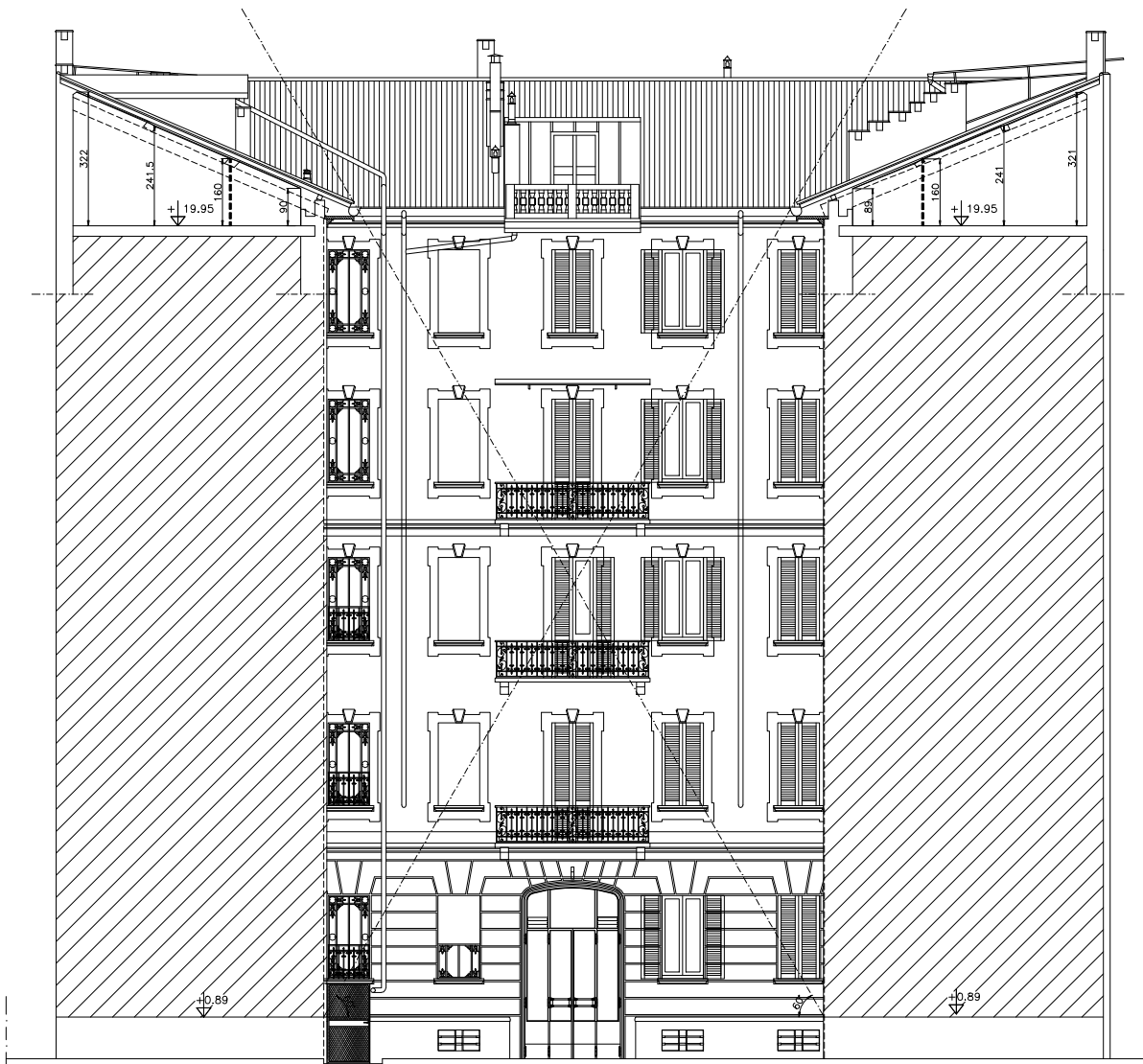
PROSPETTO D-D
